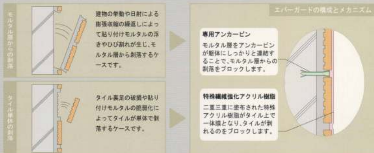
上図は下地モルタル層がある場合の構成図です
